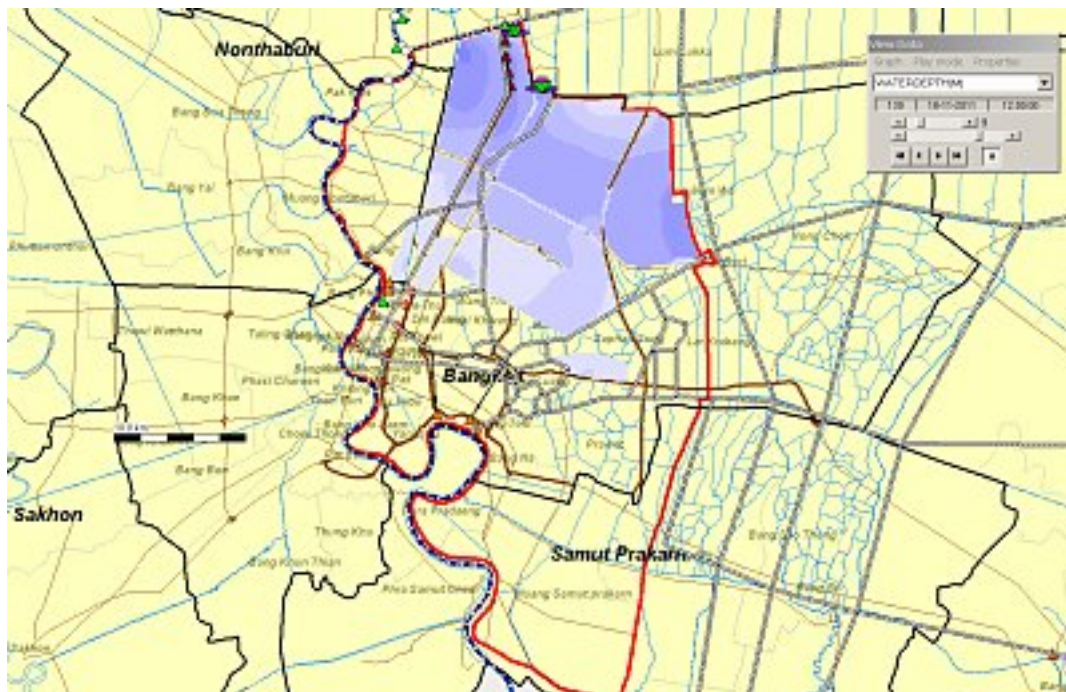
Het overstromingsmodel voor Bangkok dat in Delft werd ontwikkeld
